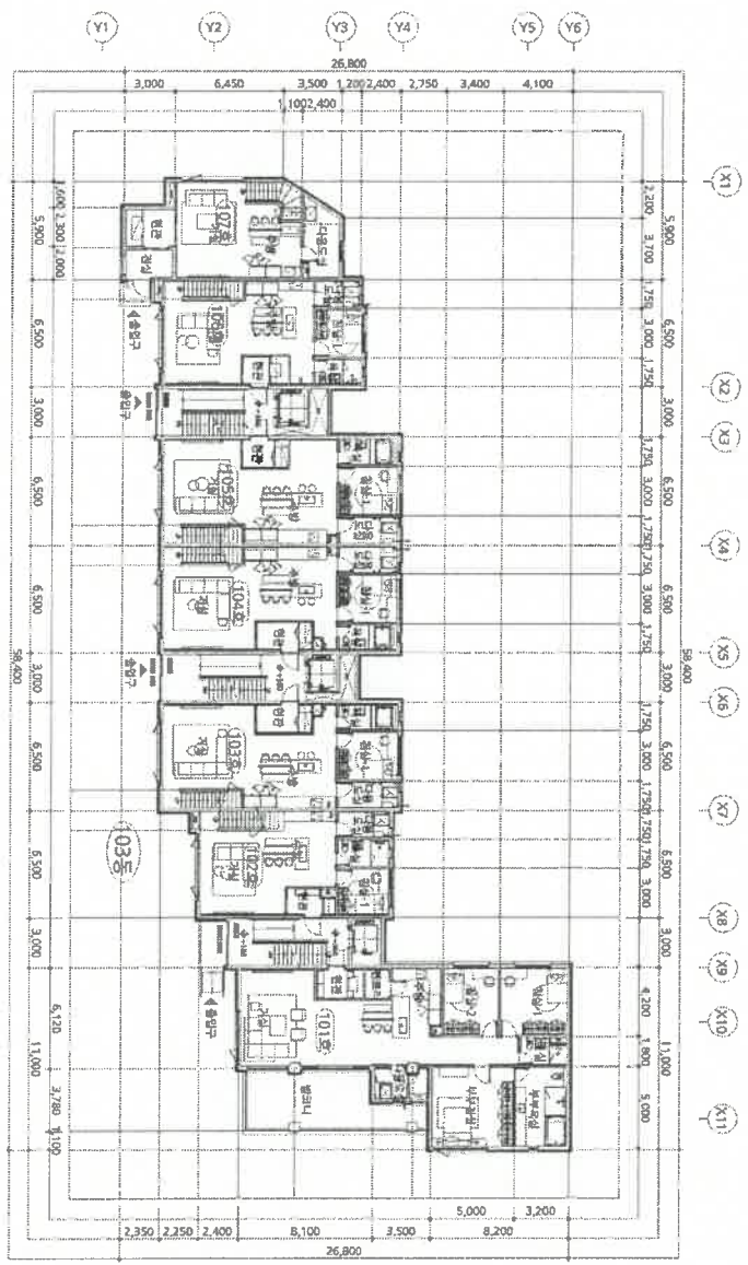
103동 1층 평면도
