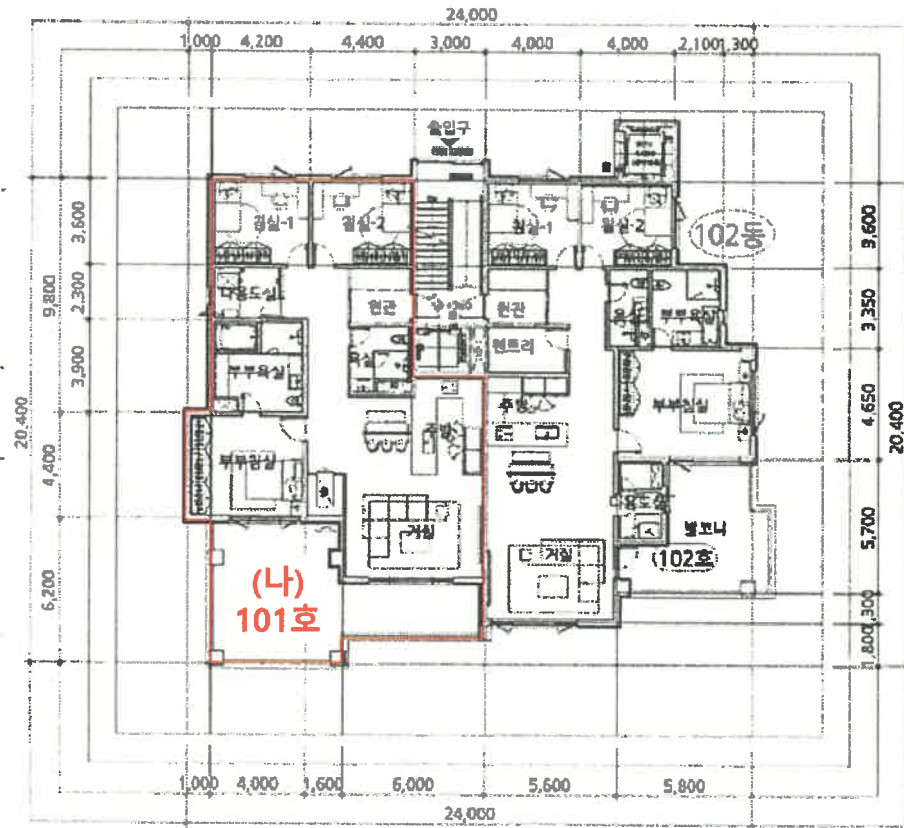
[호별배치도]
