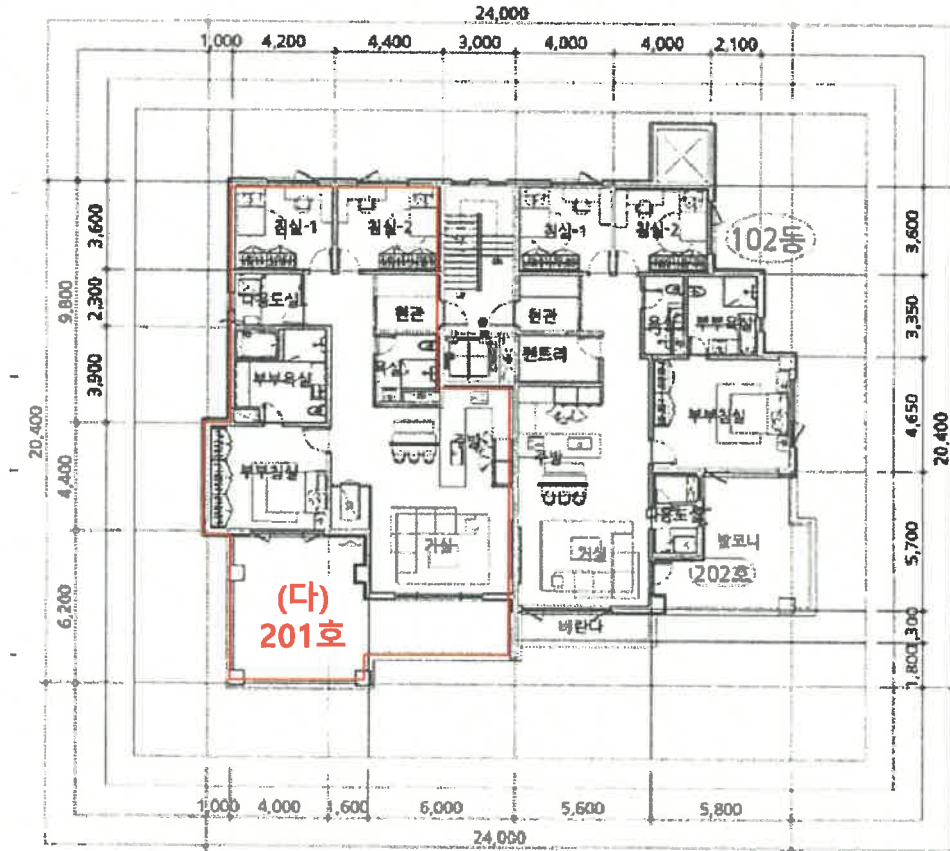
[호별배치도]
