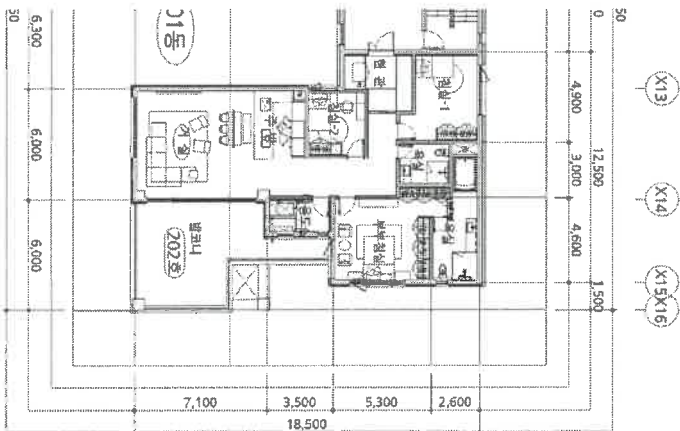
101동 2층 202호 평면도
