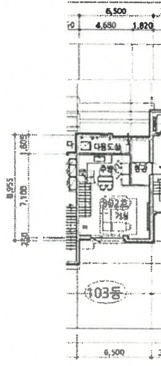
(나) 103동 302호 4층 부분
