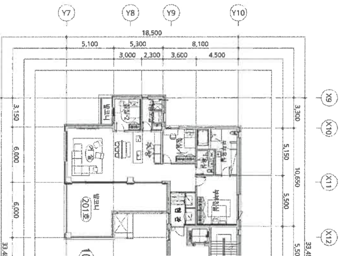
101동 2층 201호 평면도
