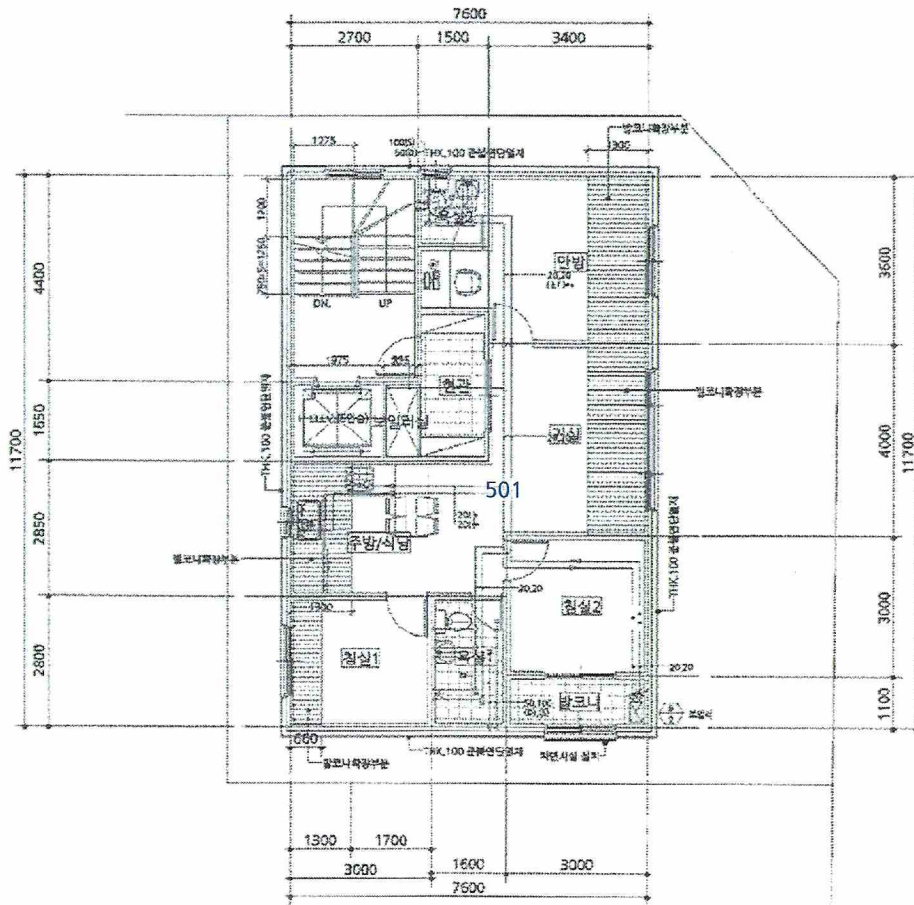
가) 5층 (공부상 면적 : 70.19㎡)
