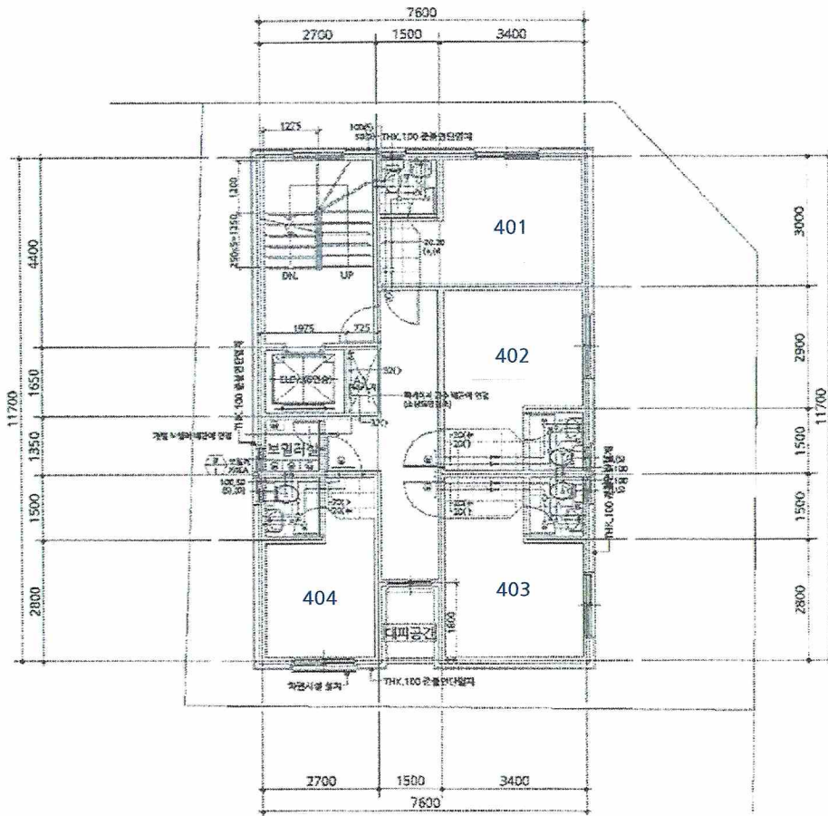
가) 4층 (공부상 면적 : 84.33㎡)
