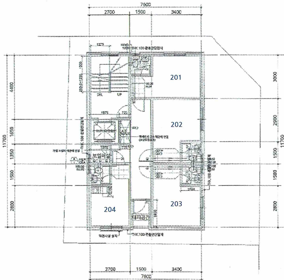
가) 2층 (공부상 면적 : 84.33㎡)
