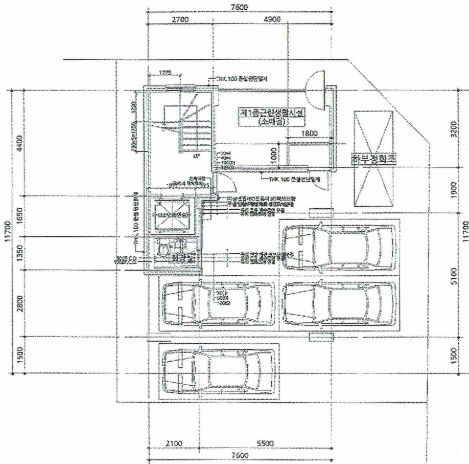
가) 1층 (공부상 면적 : 33.65㎡)
